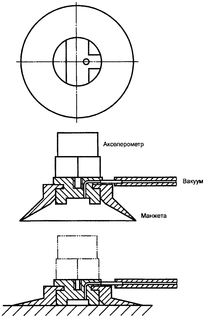
Рисунок 11 — Вакуумное крепление
