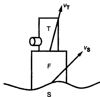
Рисунок 1 — Схематическое изображение установки акселерометра
